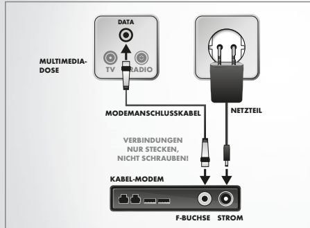
Einsatzmöglichkeit des Kabels bei Multimediodosen
